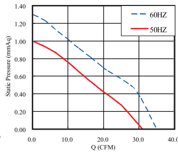
JE-03019A
