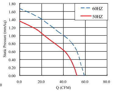
JE-03029A
