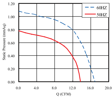
JE-03009A
