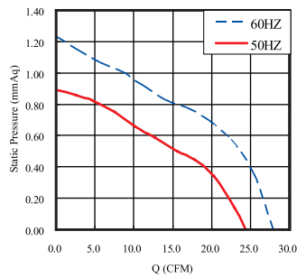
JE-03015A
